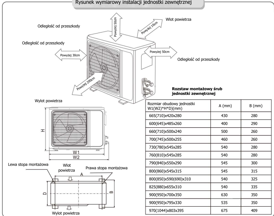
Rysunek wymiarowy instalacji jednostki zewnętrznej
